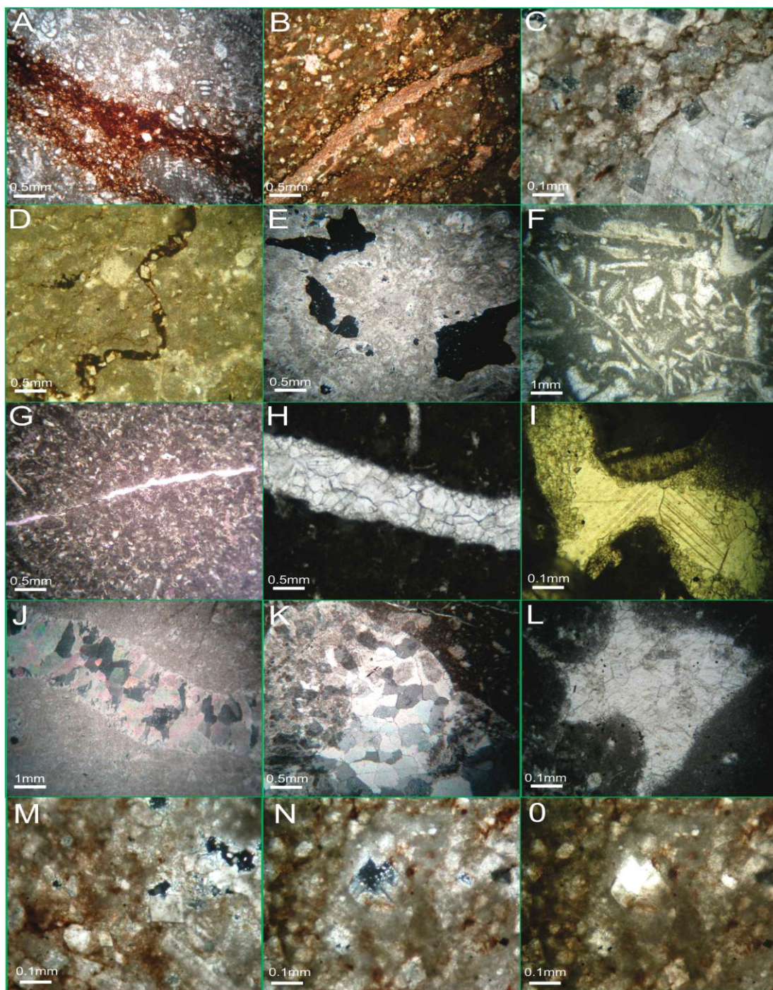
شکل ۶- برخی از مهمترین عوارض دیاژنزی مشاهده شده در کربنات‌های سروک در میدان مورد مطالعه. D-A: دولومیتی شدن و استیلولیتی شدن همراه با آن (به روابط بافتی توجه کنید)، E: انحلال فراگیر (غالباً تلوزنتیک)، F: انحلال انتخاب کننده فابریک (غالباً متوریک)، G: شکستگی باز، H: شکستگی بسته شده با سیمان، I-L: سیمان‌های دفنی نیمه عمیق تا عمیق، M-O: دولومیت‌های حل شده و بعضاً کلسیتی شده که قالب آنها حفظ شده است.
