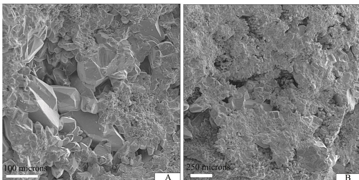
شکل ۶- حضور سیمن‌های کلسیتی درشت در مطالعات میکروسکوپ الکترونی مشخص است. این سیمن‌ها هم به صورت بین‌دانه‌ای (A) و هم به صورت هم‌ضخامت (B) مشخص هستند.
