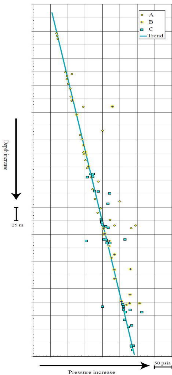
شکل ۹- روند تغییرات فشارهای اولیه سازند در مخازن کنگان و دالان در سه چاه مورد مطالعه
