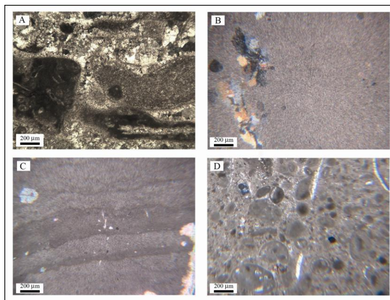
شکل ۳- رخساره‌های پس از مرز انقراض. رخساره گریستون اینتراکلاستی / آئیدی (A)، رخساره مادتون با تبخیری‌ها (B)، رخساره باندستون استروماتولیتی (C)، رخساره پکستون-وکستون پلوئیدی-انکوئیدی (D)
