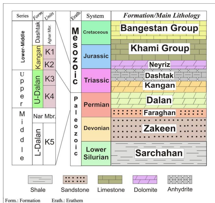
شکل ۱- توالی چینه‌شناسی سازندهای سیلورین زیرین تا کرتاسه در بخش مرکزی خلیج فارس (توکلی ۱۳۹۳)
