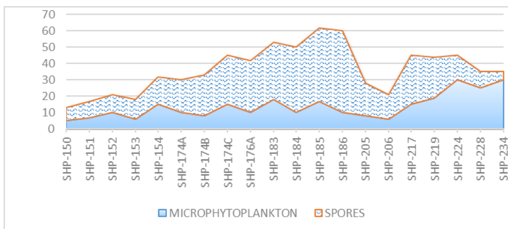
شکل ۳- فراوانی نسبی اسپورها و میکروفیتوپلانکتون‌های دریایی نمونه‌های سازند شیشتو در برش چینه‌شناسی کوه تیر، شمال غرب کرمان.
