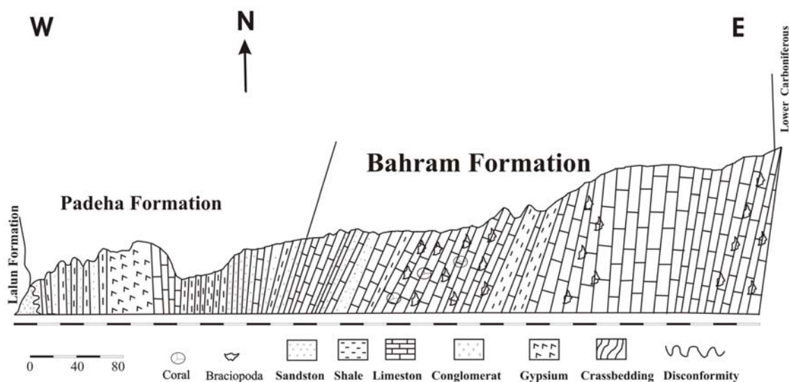
شکل ۲- نیمرخ زمین شناسی سازند پادها و بهرام در ناحیه شاهزاده محمد کرمان
