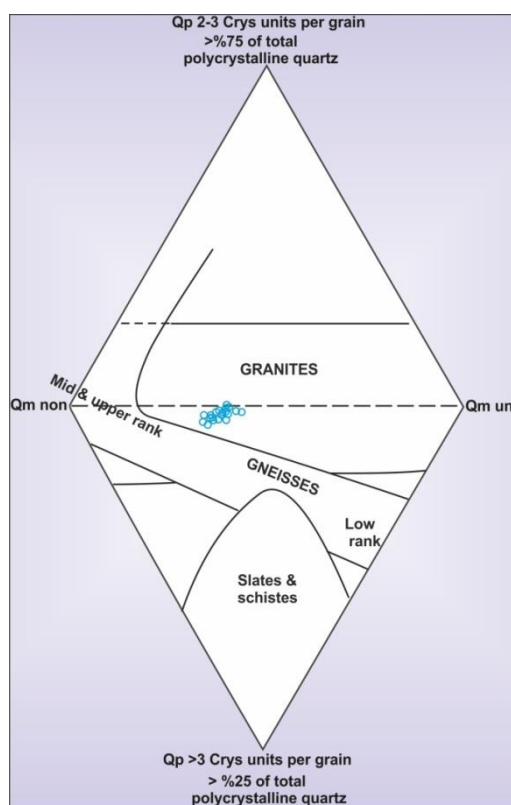
شکل ۹- نمودار تورتوزا و همکاران (Tortosa et al. 1991) به منظور تعیین منشأ ماسه‌سنگ‌های سازند پادها در برش خوش بیلاق
