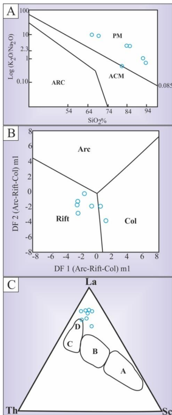
شکل ۱۲ - A. نمودار محتوای \text{SiO}_2 در برابر \text{K}_2\text{O}/\text{Na}_2\text{O} (Roser and Korsch 1986)؛ ماسه‌سنگ‌های سازند پادها در محدوده حاشیه غیرفعال قاره‌ای قرار گرفته‌اند، B. نمودار تفکیکی ورما و آرمسترانگ (Verma and Armstrong-Altrin 2013) برای تفکیک جایگاه‌های تکتونیکی ریف‌تی، برخوردی و کمان ولکانیکی، C. نمودار مثلثی Th-La-Sc (Bhatia and Crook 1986) که جایگاه تکتونیکی غیرفعال قاره‌ای را برای ماسه‌سنگ‌های سازند پادها نشان می‌دهد. نشانه‌های اختصاری در شکل: A: جزایر کمانی اقیانوسی، B: جزایر کمانی قاره‌ای، C: حاشیه فعال قاره‌ای، D: حاشیه غیرفعال قاره‌ای
