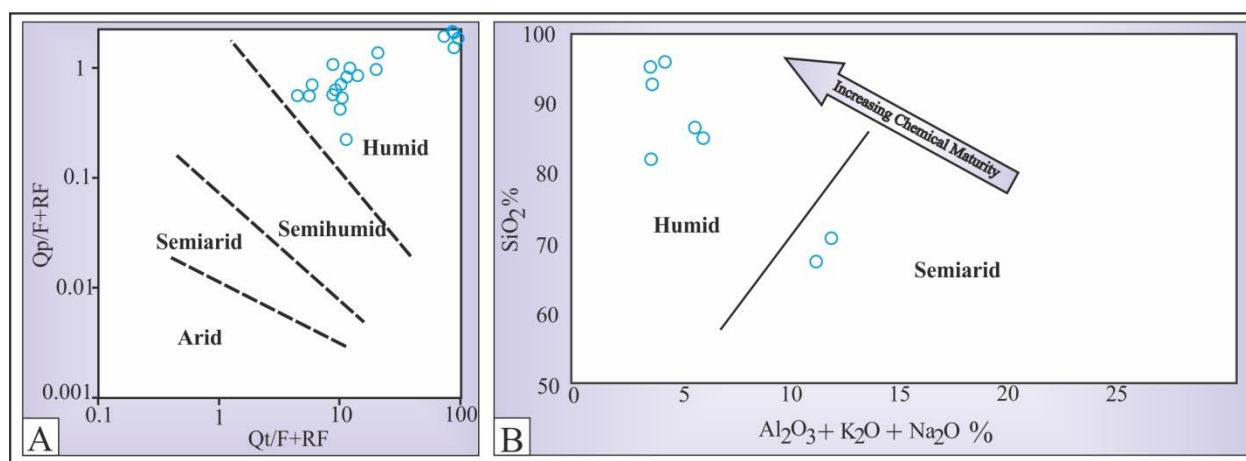
شکل ۸- A. نمودار تغییرات نمایی \text{Qt}/(\text{F}+\text{RF}) و \text{Qp}/(\text{F}+\text{RF}) (Suttner and Dutta 1986). بر اساس این نمودار، داده‌های حاصل از نقطه‌شماری ماسه‌سنگ پادها در محدوده آب‌وهوای مرطوب قرار می‌گیرند. B. نمودار دوتایی \text{SiO}_2 در برابر مجموع \text{Al}_2\text{O}_3 + \text{K}_2\text{O} + \text{Na}_2\text{O} ساتنر و دوتا (Suttner and Dutta 1986) برای تعیین وضعیت آب‌وهوای دیرینه
