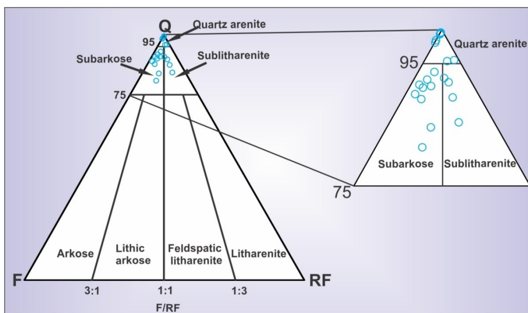
شکل ۶- نمودار مثلثی فولک (Folk 1980) به منظور طبقه‌بندی نمونه‌های ماسه‌سنگی سازند پادها در برش خوش بیلاق
