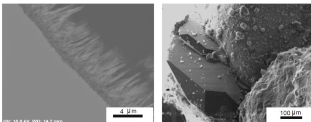
شکل ۶- تصاویر پتروگرافی کانی رسی کلریت با شکل پوشاننده ذرات در ماسه‌سنگ‌های کرتاسه بالایی سازند تاسکولوسا در کشور آمریکا؛ الف. تصویر میکروسکوپ الکترونی (SEM) تشکیل سیمان کوارتزی در محل‌هایی را نشان می‌دهد که کانی رسی کلریت با شکل پوشاننده ذرات وجود ندارد، ب. تصویر الکترونی بک اسکتر (Back Scattered Electrons/BSE) بلورهای کوچک کلریت اتوژنیک را نشان می‌دهد که به شکل عمود بر سطح خارجی دانه‌های تخریبی رشد کرده‌اند (Kordi et al. 2010, 2017a).
