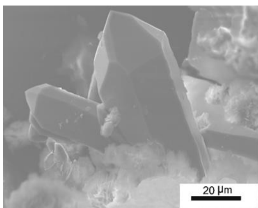
شکل ۴- تصاویر پتروگرافی سیمان‌های کوارتزی در ماسه‌سنگ‌های کامبرین- اردوئین سازند ماسه‌سنگی واحد زیرین در کشور مصر که موجب از بین رفتن تخلخل و تراوایی شده‌اند؛ الف. تصویر میکروسکوپ نوری (XPL) سیمان‌های کوارتزی با شکل رورشدی هم‌محور، ب. تصویر میکروسکوپ الکترونی (SEM) نشان‌دهنده شکل‌های یوهدرال سیمان‌های کوارتزی (Kordi et al. 2011)
