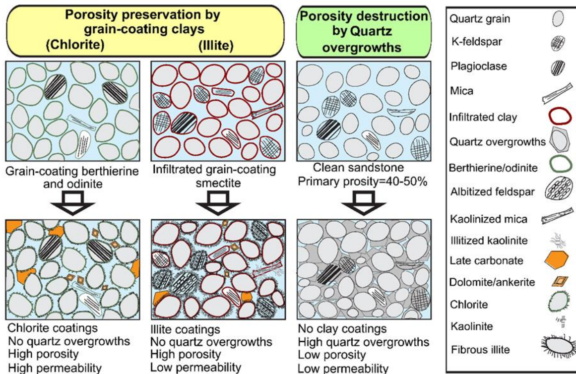
شکل ۸- طرح شماتیک نشان‌دهنده مراحل مختلف و تأثیر کانی‌های رسی اتوژنیک با شکل پوشاننده ذرات بر کیفیت مخزن (با تغییر از
