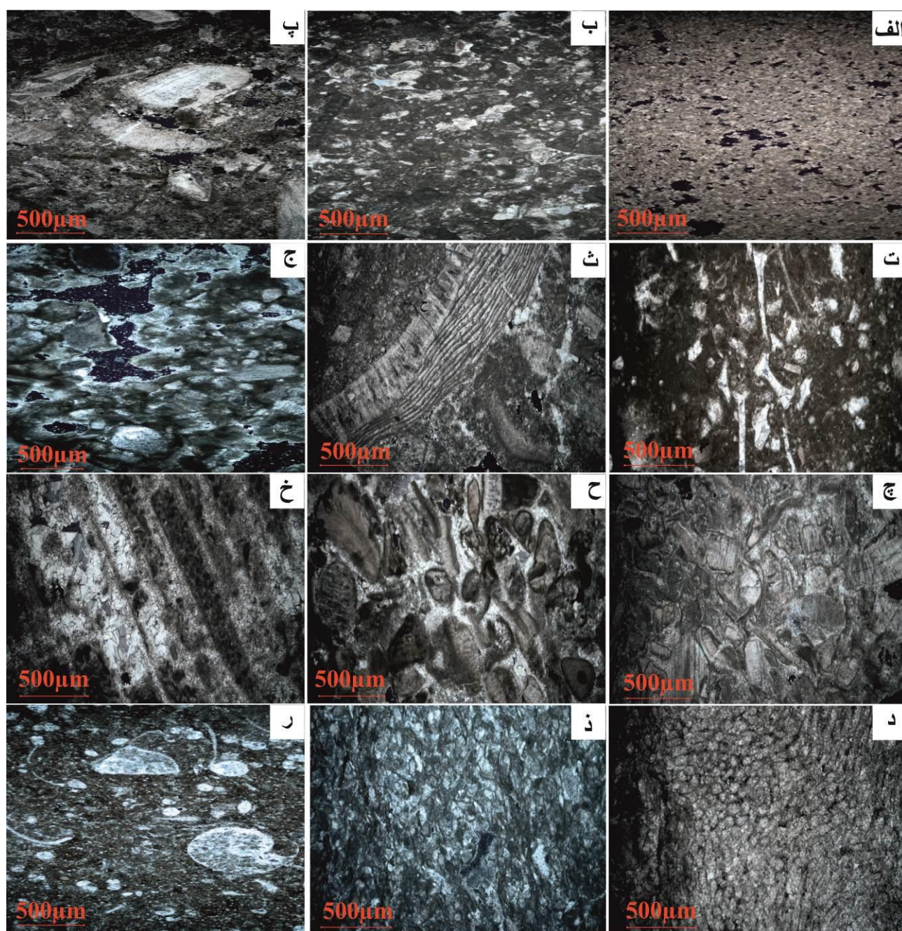
شکل ۳- الف. ریزرخساره مادستون (چاه SIE-5، عمق ۲۸۴۸)، ب. ریزرخساره وکستون تا پکستون حاوی خرده‌های اسکلتی (چاه SIE-6، عمق ۲۸۷۷)، پ. ریزرخساره وکستون تا پکستون حاوی خرده‌های اسکلتی و اینتراکلیست (چاه SIE-6، عمق ۲۸۸۱)، ت. ریزرخساره وکستون حاوی خرده‌های اسکلتی و پلوئید همراه با آشفستگی زیستی (چاه SIE-6، عمق ۲۹۰۶)، ث. ریزرخساره وکستون تا پکستون حاوی خرده‌های اسکلتی رودیست (چاه SIE-5، عمق ۲۸۵۵)، ج. ریزرخساره گرینستون حاوی خرده‌های اسکلتی و اینتراکلیست (چاه SIE-5، عمق ۲۸۷۶)، چ. ریزرخساره گرینستون حاوی خرده‌های اسکلتی (چاه SIE-5، عمق ۲۸۶۳)، ح. ریزرخساره گرینستون حاوی خرده‌های اسکلتی و کورتوئید (چاه SIE-5، عمق ۲۸۸۶)، خ. ریزرخساره باندستون مرجانی (چاه SIE-5، عمق ۲۸۵۳)، د. ریزرخساره باندستون مرجانی (چاه SIE-5، عمق ۲۸۶۲)، ذ. ریزرخساره پکستون حاوی خرده‌های اسکلتی ریزدانه (چاه SIE-5، عمق ۲۸۹۵)، ر. ریزرخساره مادستون تا وکستون حاوی خرده‌های اسکلتی (چاه SIE-5، عمق ۲۹۱۶)
