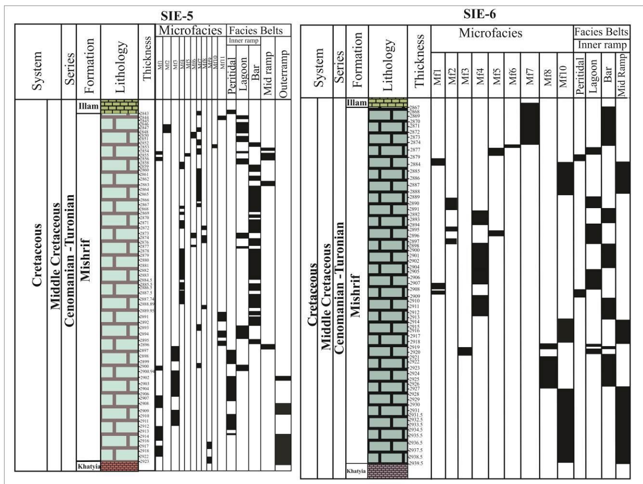
شکل ۵- ستون سنگ چینه نگاری سازند میشریف در چاه های SIE-5 و SIE-6 میدان نفتی اسفند
