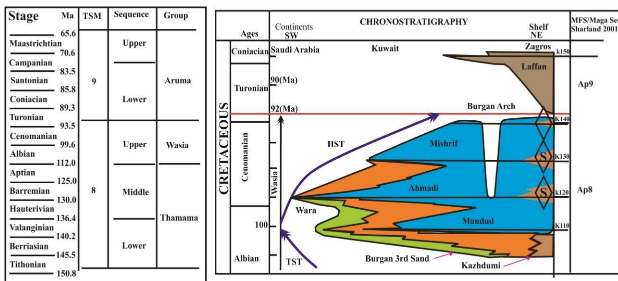
شکل ۲- توالی کروئوئاستراتیگرافی کرتاسه میانی و بالایی در صفحه عربی (Porrás and Compos 2001) همراه با اشکوب‌های کرتاسه و سن مرز میان آنها (Burchette and Britton 1985)
